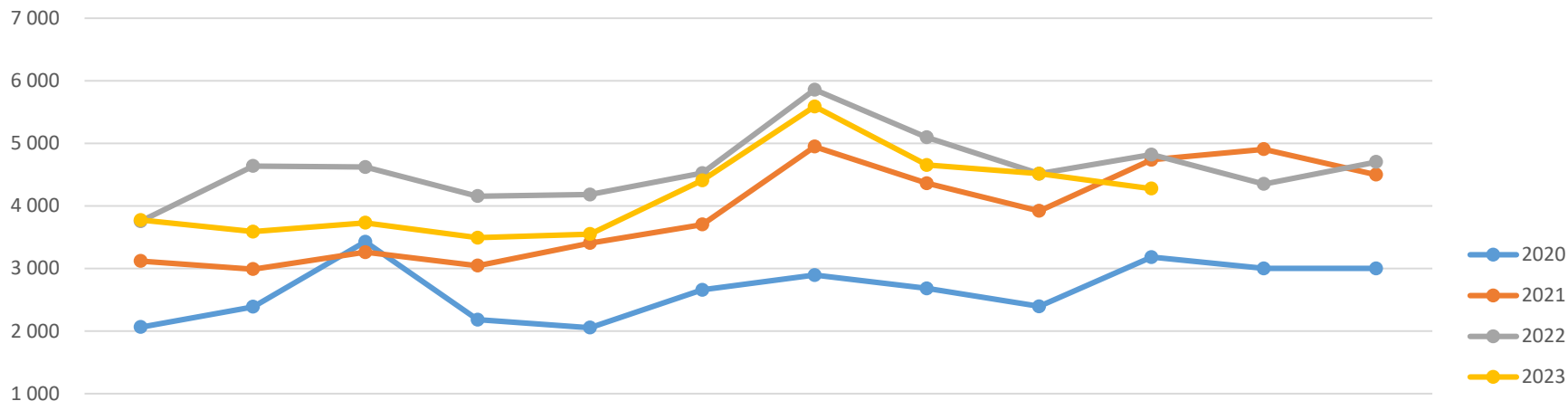
AML-trend
